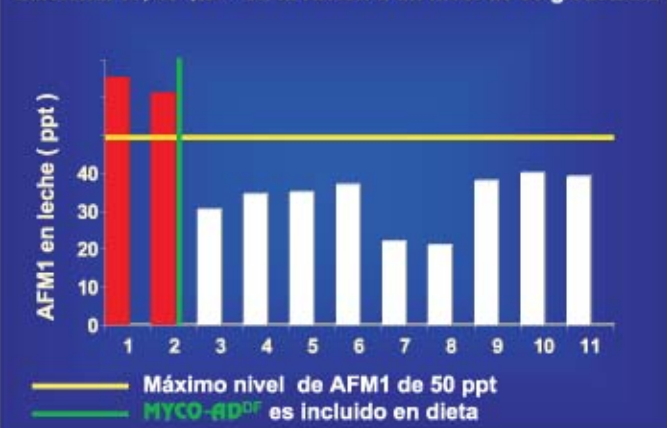
Gráfica 1. Presencia de aflatoxina M1 en la leche después de adicionar MYCO-AD DF en la ración a un nivel de 50 g/vaca/día
